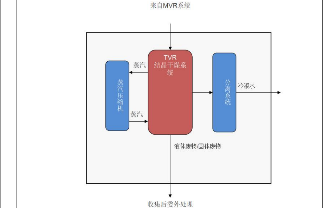
图 4-11 污水处理站 MVC 浓缩工艺流程图
