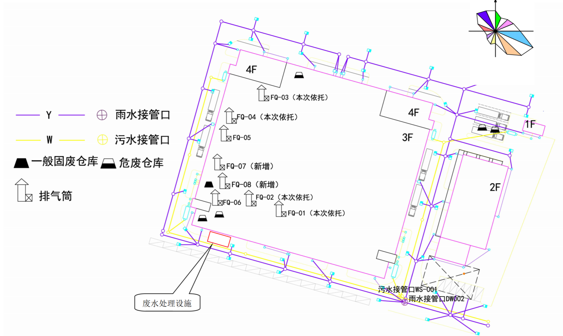
附图 4 厂区雨污水管网及平面布置图
