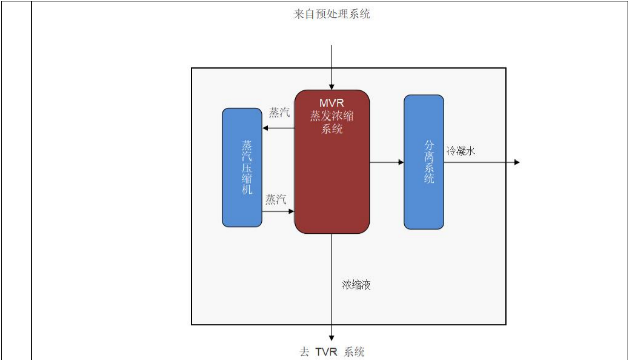
图 4-10 污水处理站 MVR 蒸发浓缩机工艺流程图
