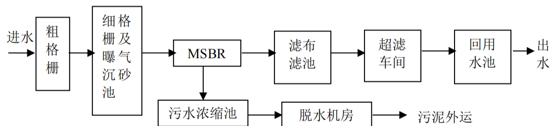
图 4-6 梅村水処理厂四期工程水處理工艺流程简图
