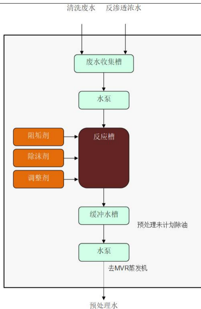
图 4-9 预处理工艺流程图
