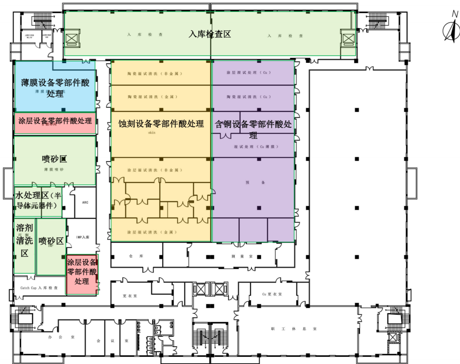
附图 5-2 2F 生产车间平面布置图
