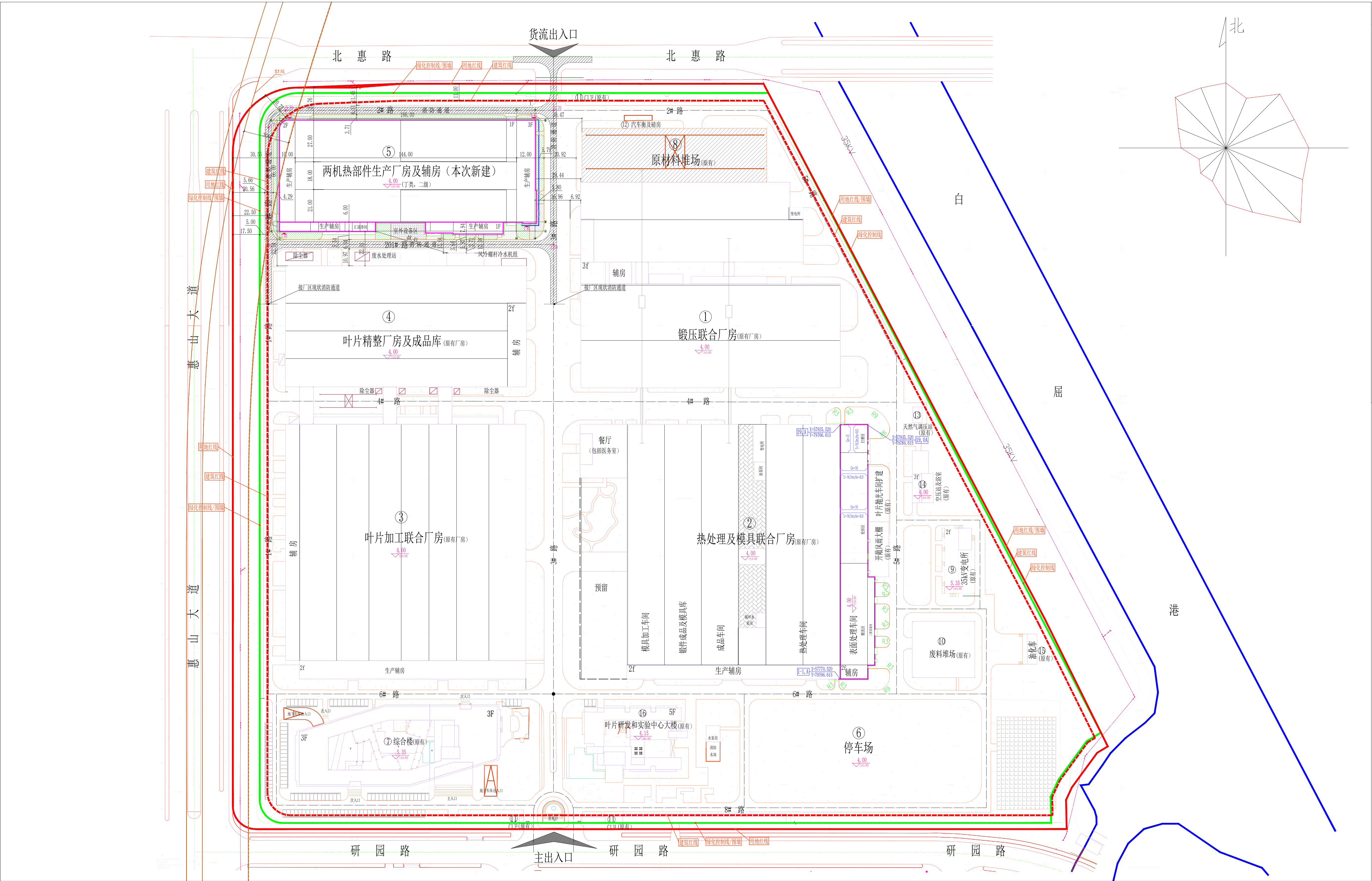
建筑总平面图 1:500
