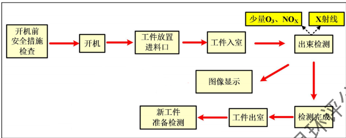
图9-6 工作流程及产污环节图
