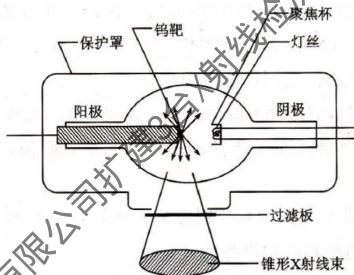
图9-5 典型的X射线管结构图
