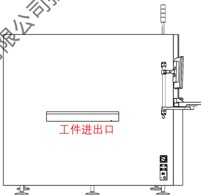
图9-2本项目X射线检测装置外部结构图（侧视）
