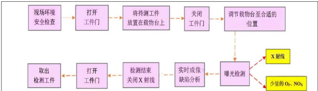
图 9-4 本项目工业 CT 装置工作流程及产污环节
