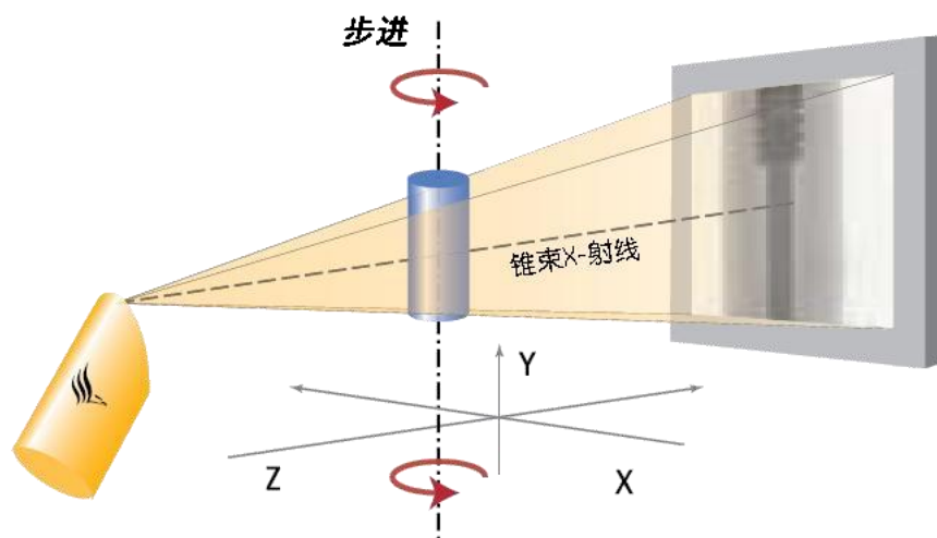
图 9-3 本项目工业 CT 装置几何示意图
