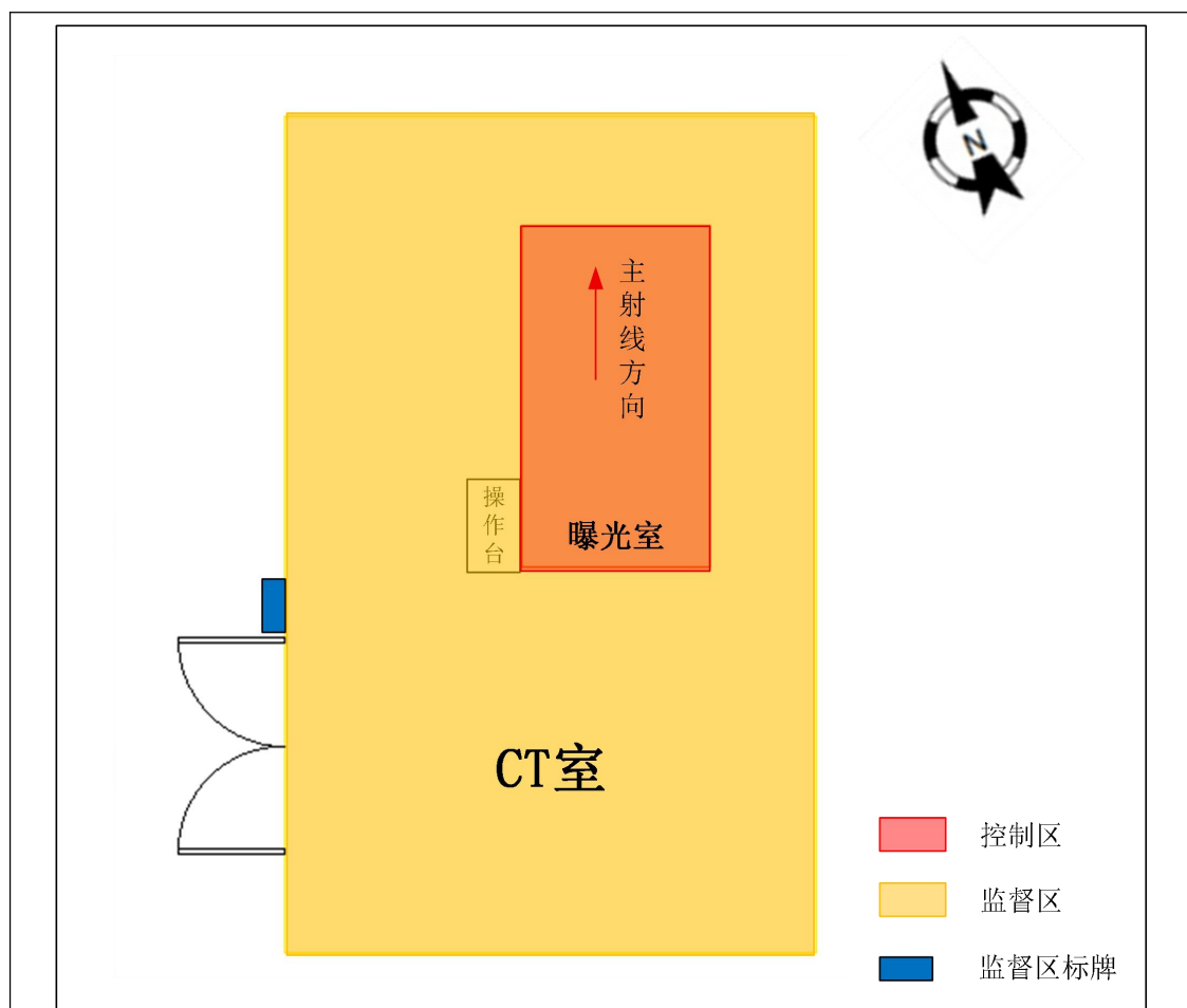
图 10-1 本项目工业 CT 装置监督区及控制区示意图
