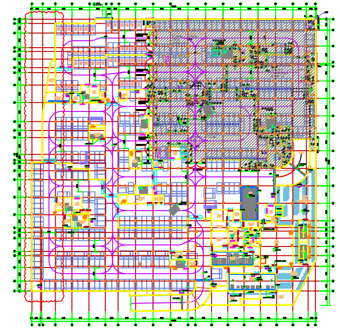
一期地下室（变更前）
