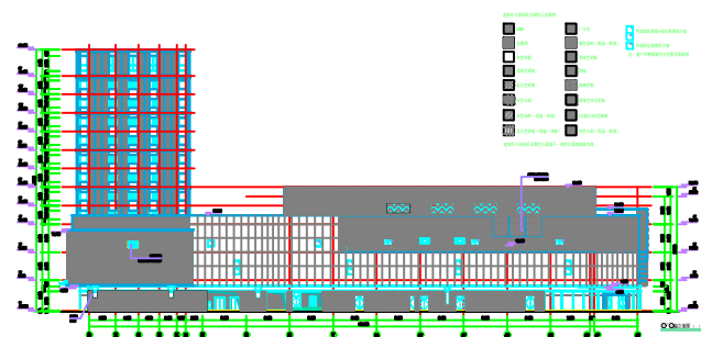
立面图（变更后）
