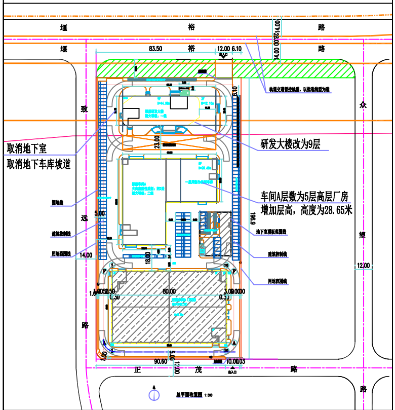
总平面图（变更后）
