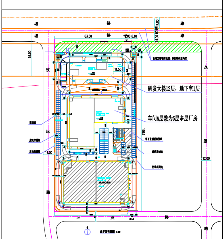
总平面图（变更后）
