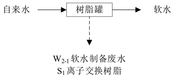
图 2-4 软水制备工艺及产污环节图
