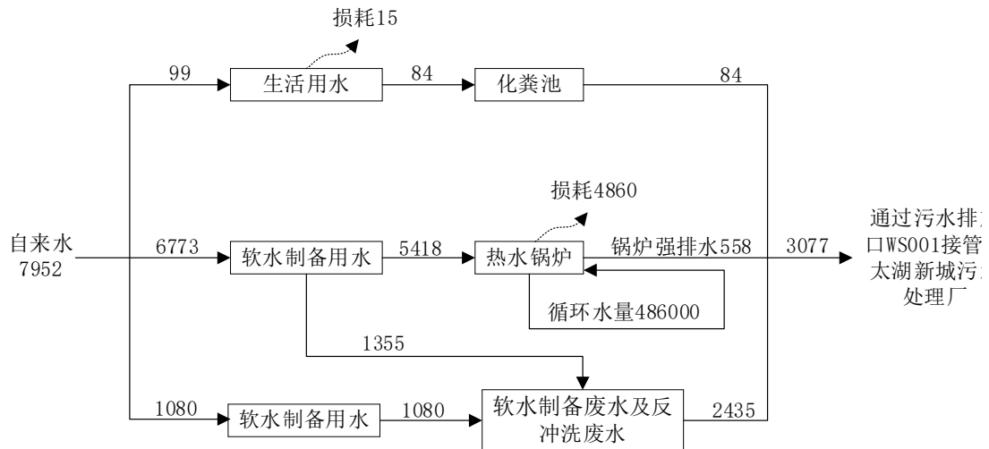
图 2-1 本项目水量平衡图（单位 t/a）
