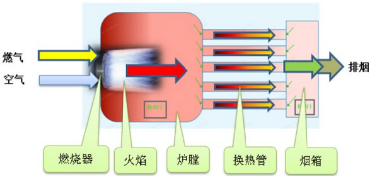
图 2-3 热水锅炉工作原理图
