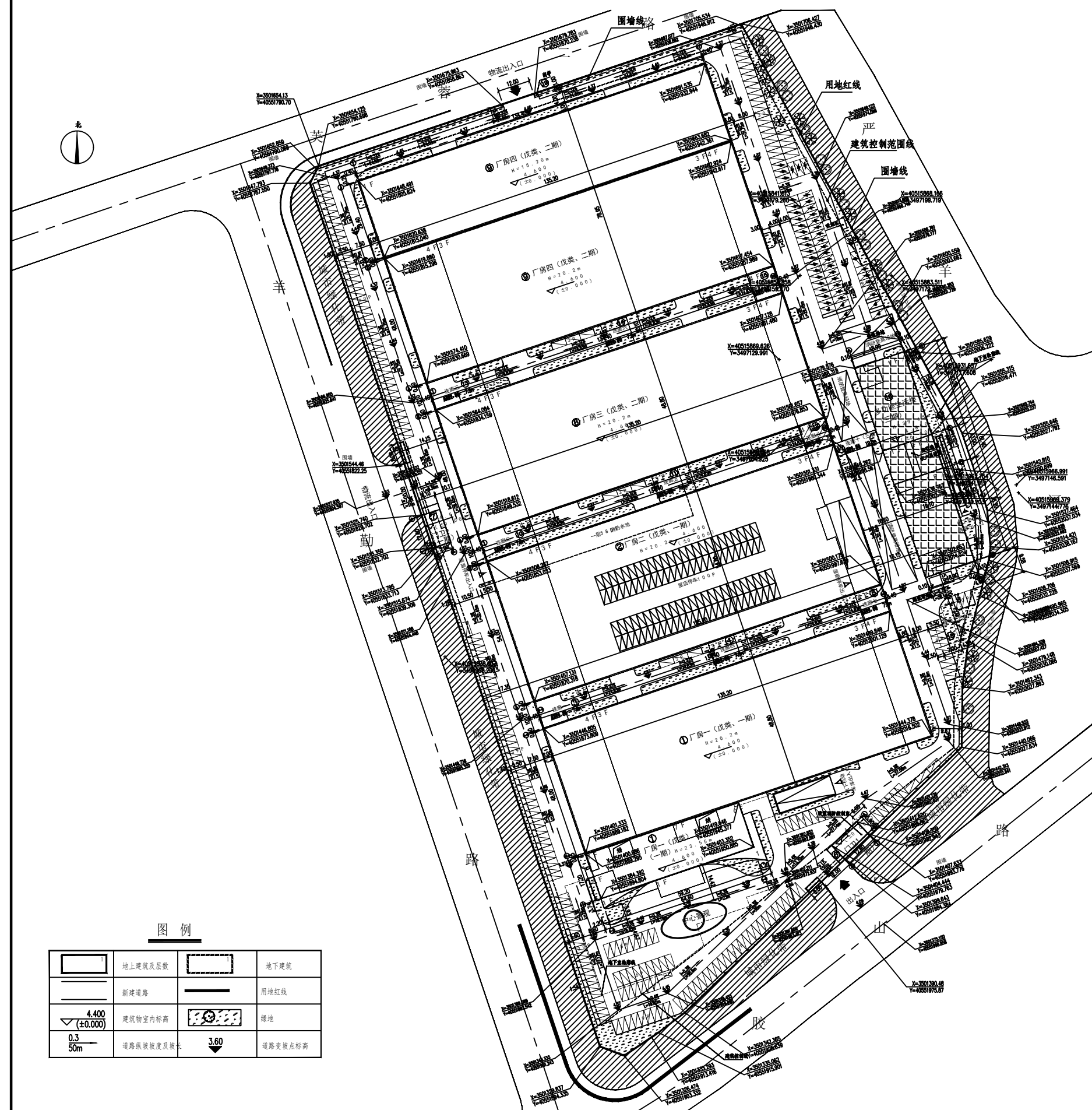
总平面布置图
