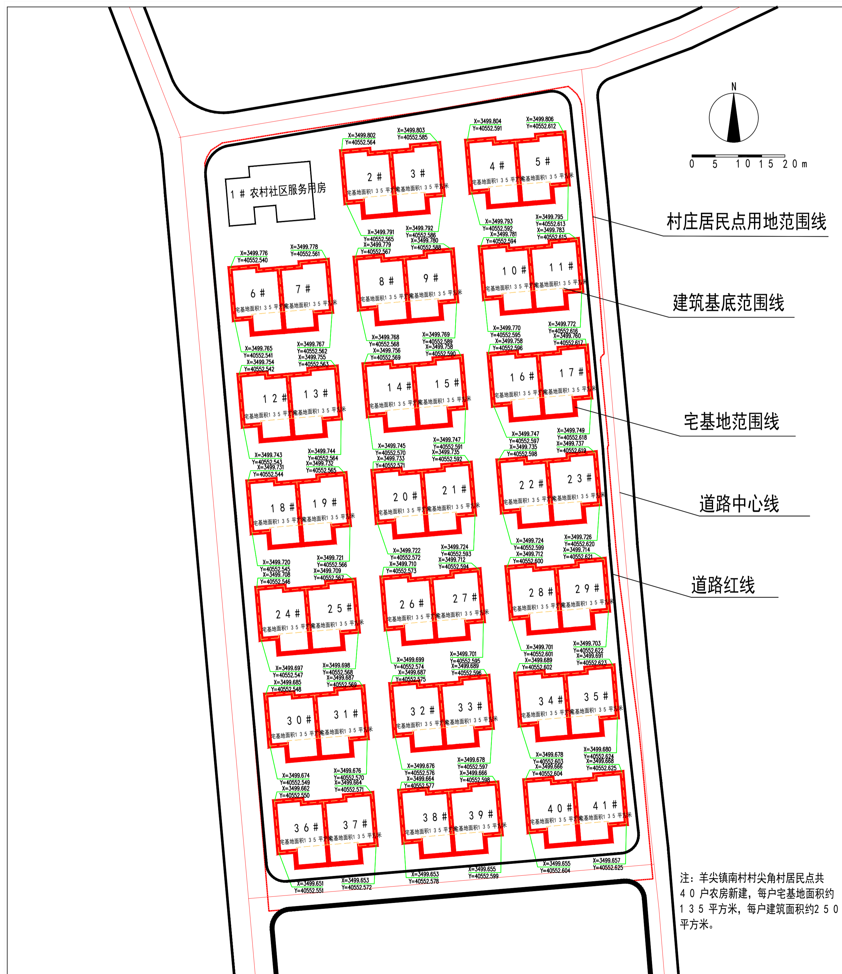
农村住房宅基地布局图
