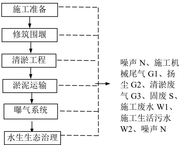
图 2-2 新开河综合整治工程施工工艺流程图
