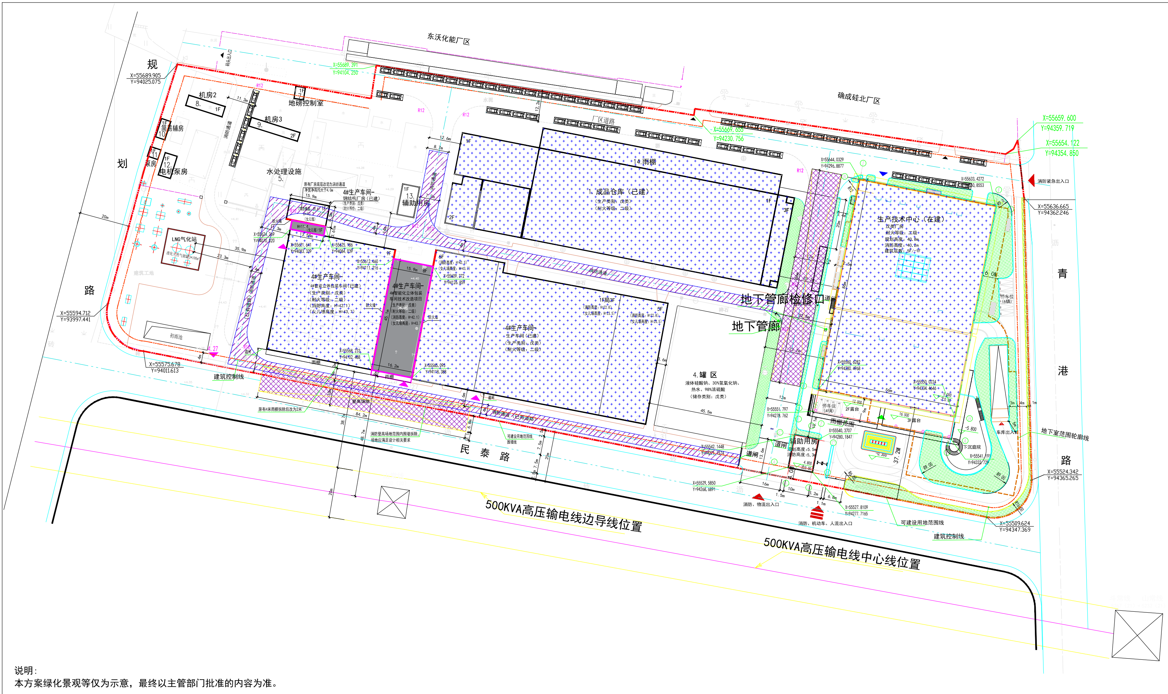
总平面图
