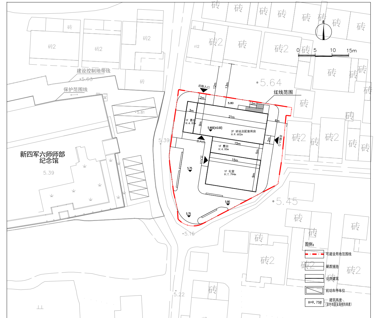
变更后方案总平面图
