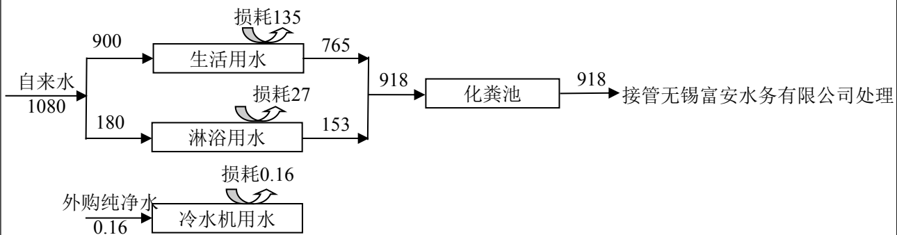
图 2-1 本项目水量平衡图 单位：t/a
